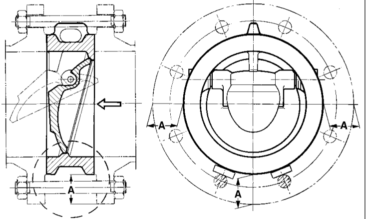
Fig. 1 Montage correct
