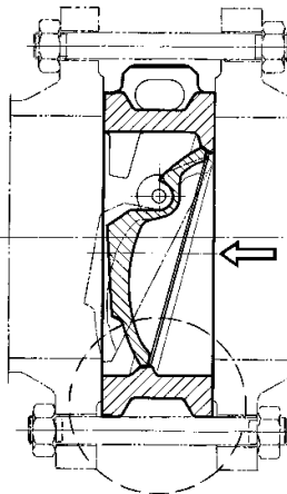
Fig. 3 Montage défectueux
