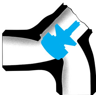
Y Angle Globe
