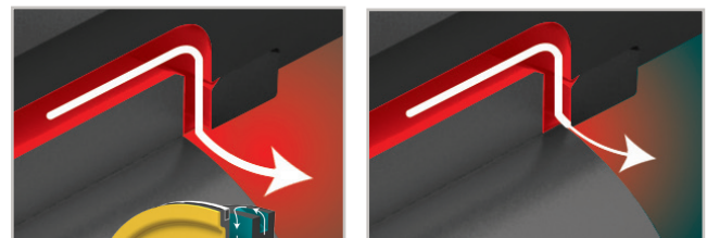
El orificio variable se abre y cierra para controlar dinámicamente la presión de la cámara de balanceo.
